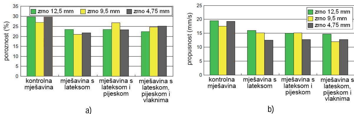
Slika 4 - Utjecaj dodatka i veličine agregata na: a) poroznost; b) propusnost, [10] (sliku uredili autori)
