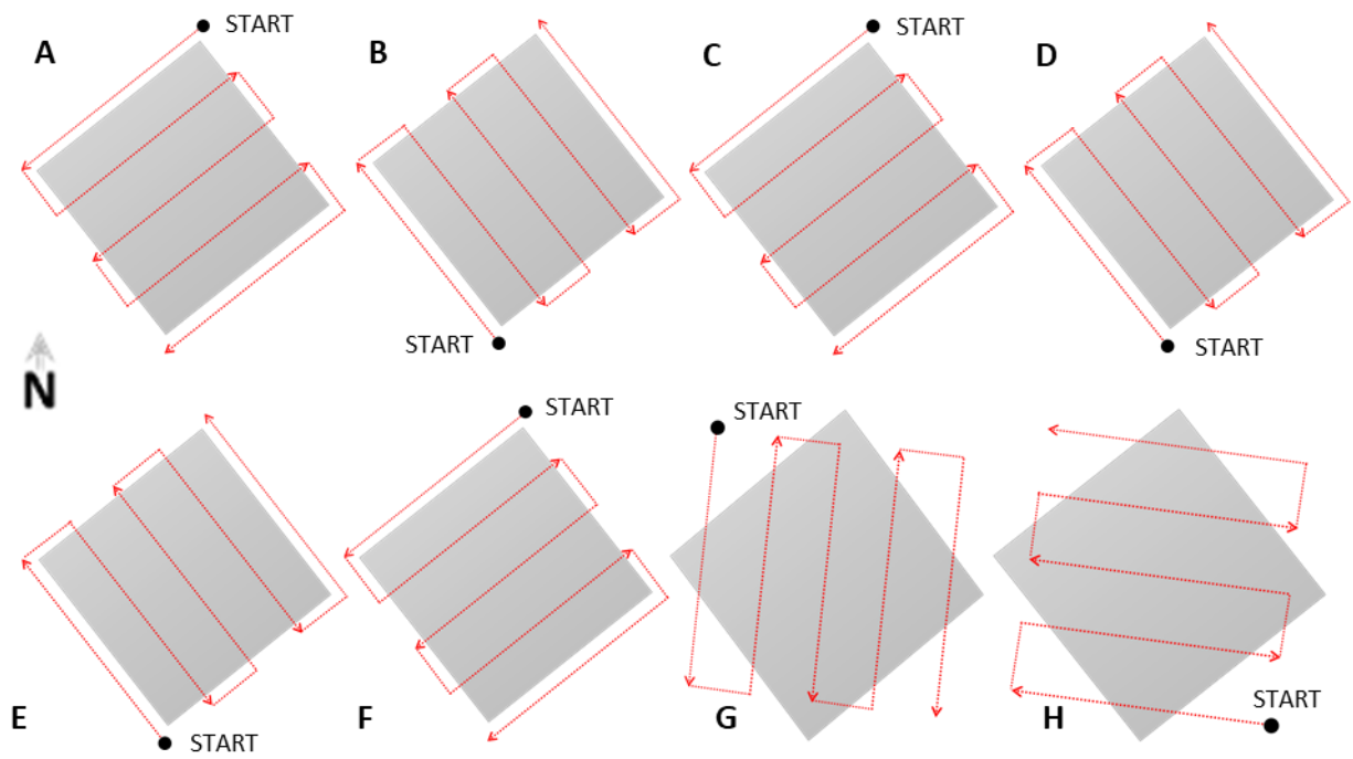
Slika 30. Izvedeni scenariji MBES snimanja odabrane testne plohe
