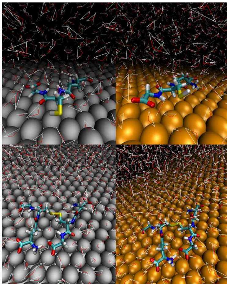
Slika 40. Posljednji kadrovi produkcijske faze molekulske dinamičke simulacije: GSH na površini Ag (gore lijevo) ili Au (gore desno), GSSG na površini Ag (dolje lijevo) ili Au (dolje desno). GSH i GSSG prikazani su modelom kugle i štapića jednakog promjera. Ag i Au prikazani su kalotnim modelom u sivoj, odnosno narančastoj boji. Molekule vode prikazane su linijskim/ žičanim prikazom.
