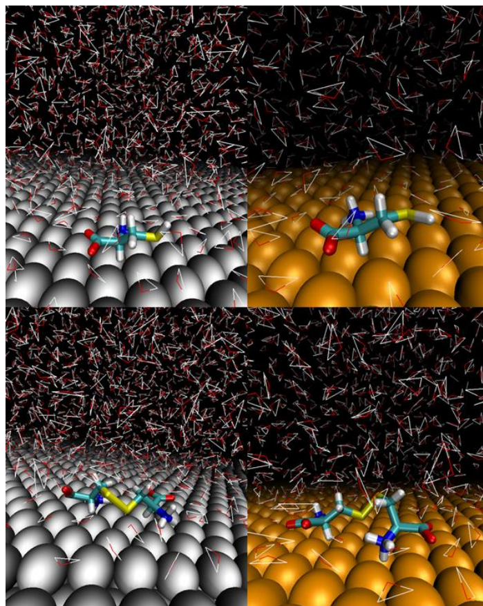
Slika 39. Posljednji kadrovi produkcijske faze molekulske dinamičkih simulacija: CYS na površini Ag (gore lijevo) ili Au (gore desno), cistina na površini Ag (dolje lijevo) ili Au (dolje desno). CYS i cistin prikazani su modelom kugle i štapića jednakog promjera. Ag i Au prikazani su kalotnim modelom u sivoj, odnosno narančastoj boji. Molekule vode prikazane su linijskim/ žičanim prikazom.
