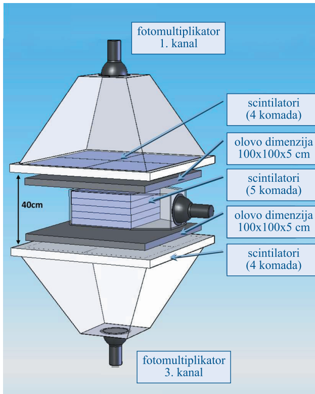
Sl. 6.: Shematski prikaz detektora SEVAN
