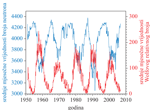
Sl. 3.: Tok kozmičkog zračenja (plava crta) antikoleriran je sa Sunčevom aktivnošću. Podaci o toku kozmičkog zračenja dobiveni su neutronske detektorom Climax Sveučilišta u Chicagu (riječ je o srednjim mjesečnim iznosima podijeljenim sa sto), dok je Sunčeva aktivnost iskazana srednjim mjesečnim iznosima Wolfova relativnog broja pjega
