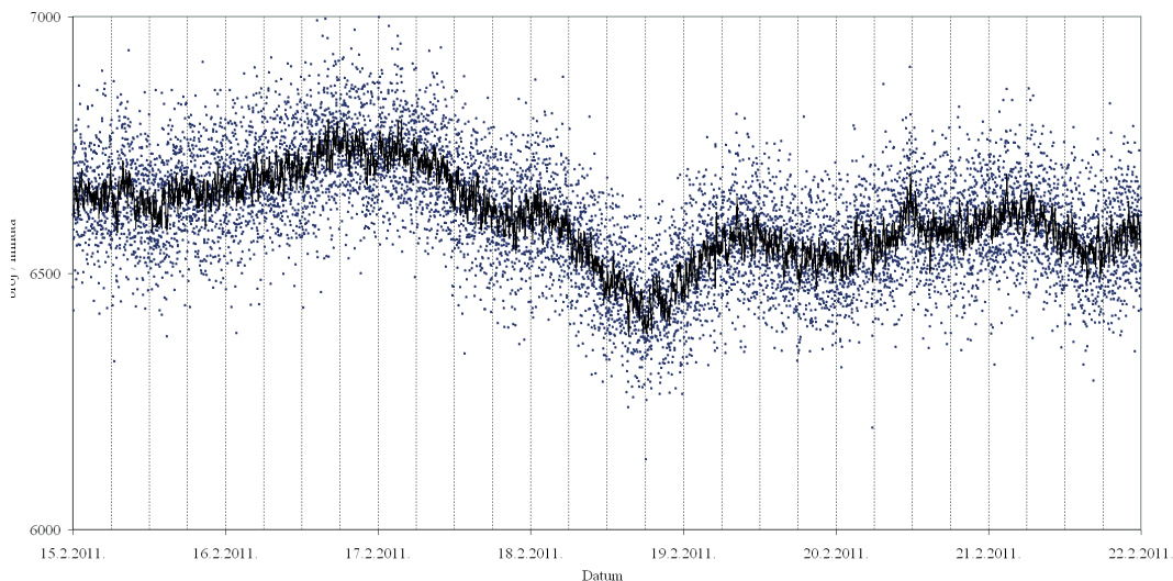
Sl. 8.: Forbushov učinak na niskoenergetske čestice detektora SEVAN CRO. Mjerenja od 17. do 18. veljače 2011. godine
