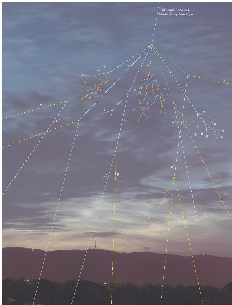
Sl. 1.: Pri interakciji primarne čestice kozmičkog zračenja s jezgrama atmosferskih atoma većinu nastalih čestica čine pioni ( p ). Neutralni pioni brzo se raspadaju (za oko 10^{-16} s), obično u dva g-fotona. Gama-fotoni mogu producirati parove elektron-pozitron, od kojih zakročnim zračenjem opet mogu nastati novi g-fotoni. Nabijeni pioni imaju dulje vrijeme raspada (oko 10^{-8} s), pa prije raspada mogu stupiti u interakciju s jezgrama drugih elementa. Pozitivno nabijeni pioni obično se raspadaju na pozitivne mione ( m ) i mionske neutrine ( n ), dok se negativni pioni obično raspadaju na negativne mione i mionske antineutrone. Negativni mioni raspadaju se stvarajući elektrone i elektronske antineutrone i mionske neutrine, dok pri raspadu pozitivnih miona nastaju pozitroni, elektronski neutrini i mionski antineutrini.. Kaskadni procesi šire se vrlo brzo u atmosferi, brzinom usporedivom s brzinom svjetlosti.
