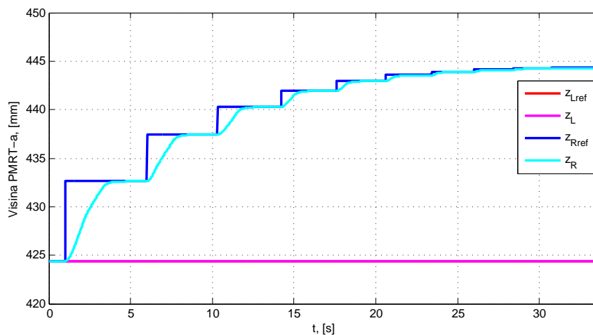
Slika 6.22: Scenarij 2: referentna visina lijevog PMRT-a ( z_{Lref} ) i desnog PMRT-a ( z_{Rref} ), trenutna visina lijevog PMRT-a ( z_L ) i desnog PMRT-a ( z_R )
