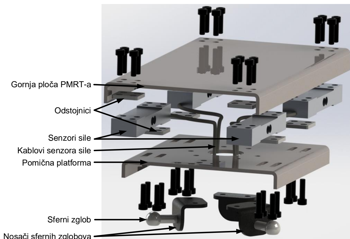
Slika 7.5: Pomična platforma paralelnog manipulatora 3-RPS s PMRT-om
