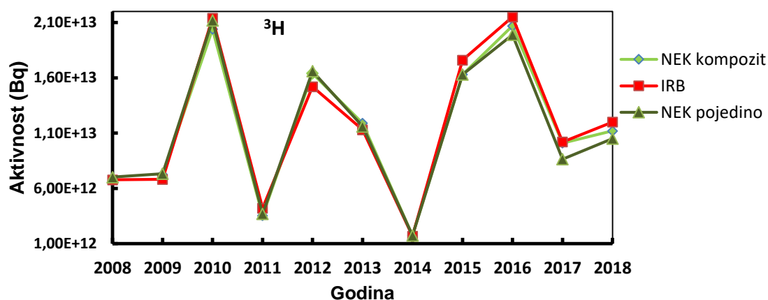
Slika 1. Usporedba rezultata mjerenja godišnje ukupne ispuštene aktivnosti ^3\text{H} iz WMT-a dobivene kao umnožak volumena ispuštene vode iz WMT i koncentracije aktivnosti tricija izmjenog u laboratorijima IRB-a i NEK-a.
