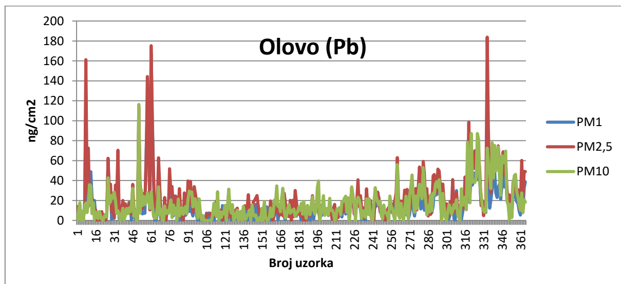
Slika 2. Prikaz koncentracija olova u lebdećim česticama aerodinamičkog promjera PM1, PM2,5 i PM10 za 2017. godinu.
