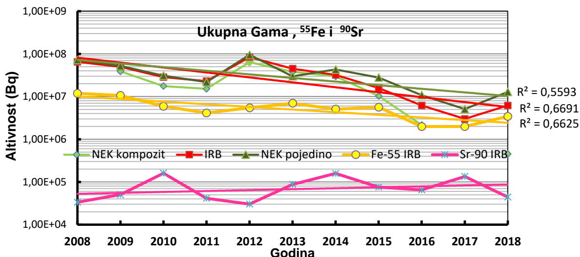
Slika 4. Usporedba mjerena ispuštene ukupne godišnje aktivnosti gama emitera te godišnje ispuštene aktivnosti ^{55}\text{Fe} i ^{90}\text{Sr} mjerene na IRB-u.
