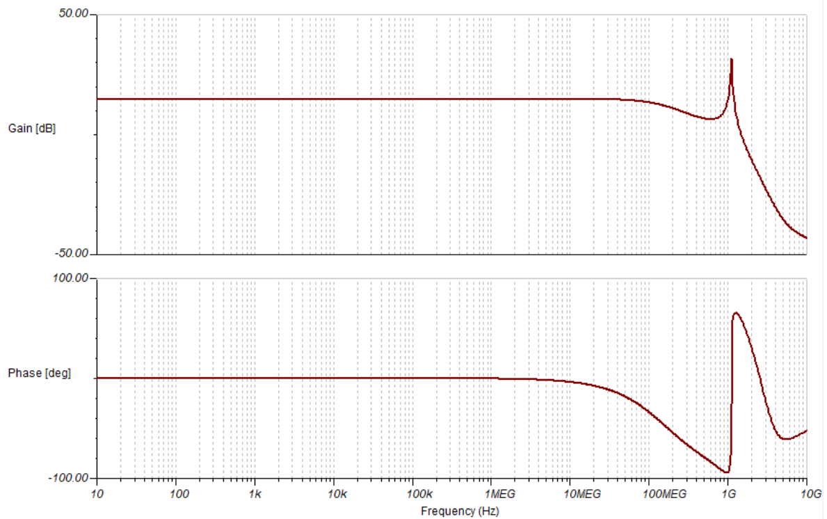
Slika 3. Bodeov dijagram frekvencijske karakteristike pojačala.
