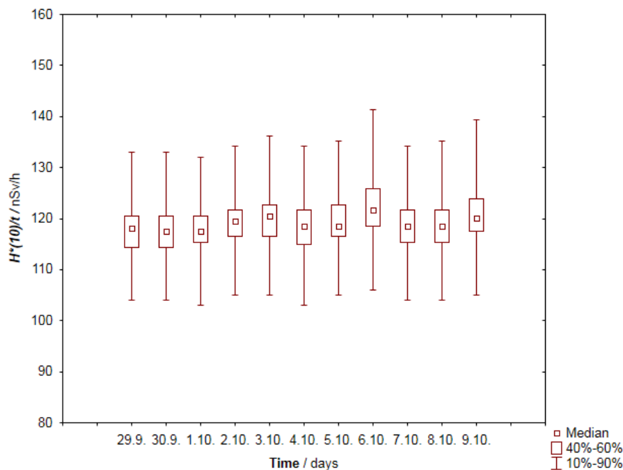
Slika 1. Medijani i raspon od 10. do 90. percentila dnevnih vrijednosti H^*(10)/t u danima potencijalnog akcidenta s ispuštanjem ^{106}\text{Ru} u prvim danima listopada 2017. godine
