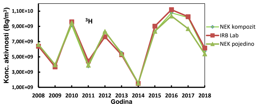
Slika 2. Usporedba rezultata mjerenja godišnje koncentracije aktivnosti ^3\text{H} u WMT-u.
