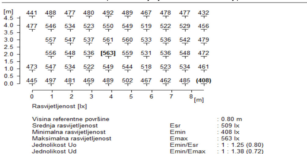
Slika 6. Tablični prikaz rasvjetljenosti na referentnoj površini
