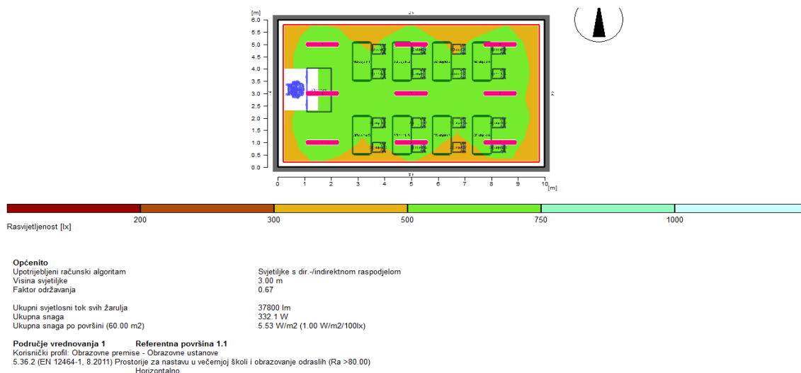
Slika 2.9: Pregled rasvjetljenosti radnog prostora svjetiljkama sa LED izvorima
