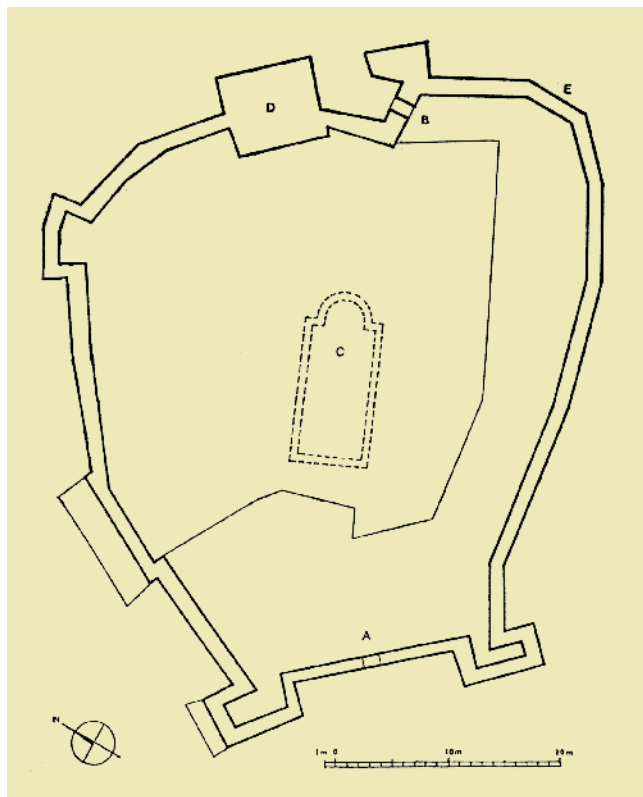
1. Tlocrt kaštela Sv. Mihovila (izvor: PETRICIOLI, I., 1987., 170.)
