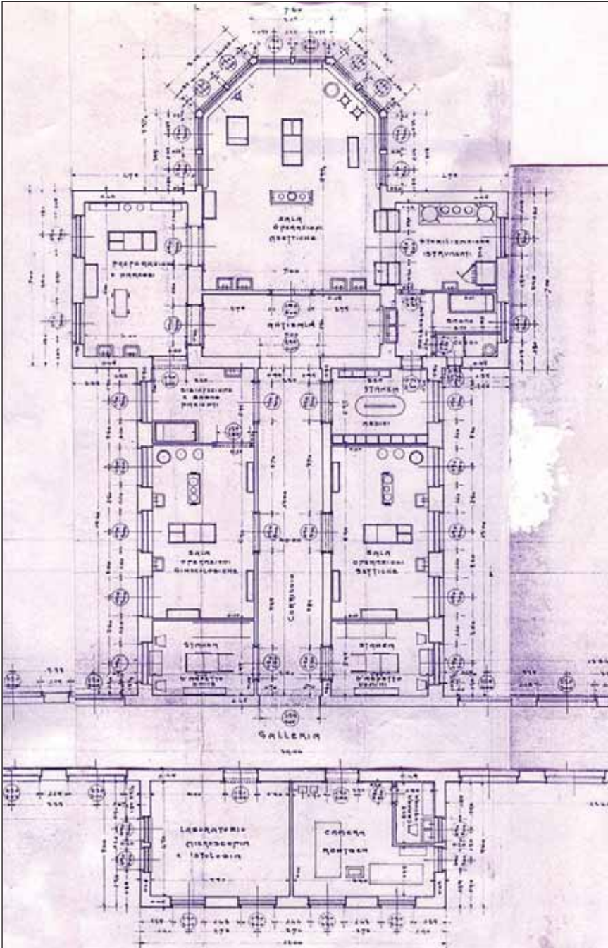
Slika 10. Projekt bolnice grada Rijeke, glavna zgrada, operacijske dvorane 2. kata Figure 10 – Rijeka city hospital, main building, operation theatres on the 2 nd floor
