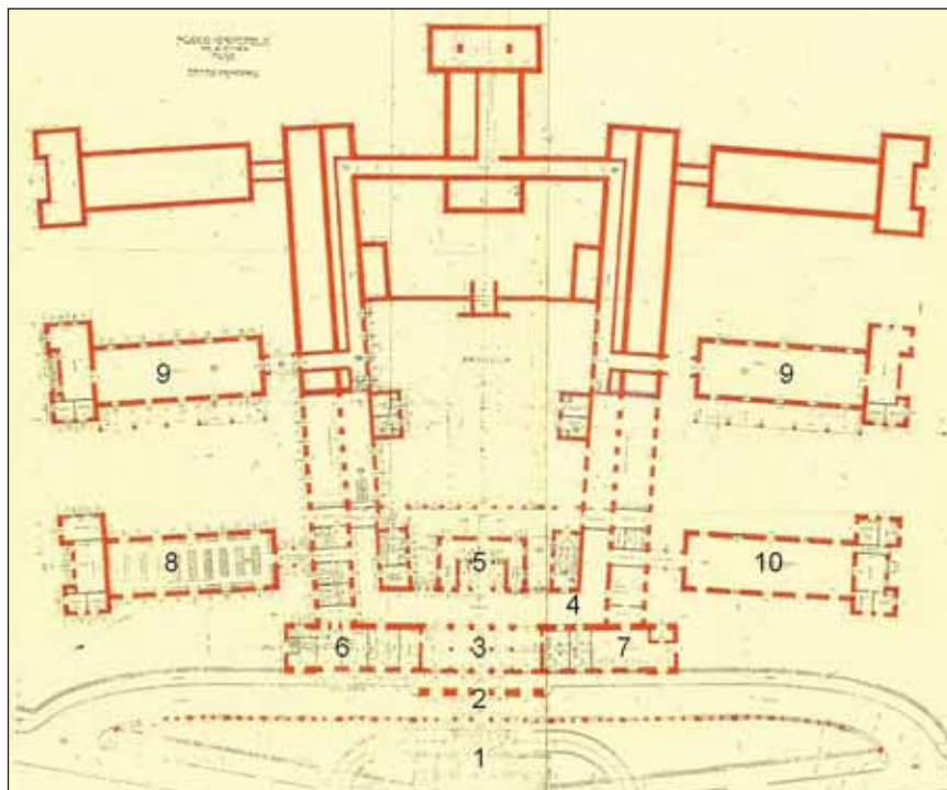
Slika 3. Projekt bolnice grada Rijeke, glavna zgrada, tlocrt prizemlja: 1. prilazno stubište, 2. trijem, 3. atrij, 4. hodnik, 5. stubište i dizala, 6. prijамni ured, 7. direktor i uprava, 8. centralna garderoba (spremište privatnih odijela), 9. spremišta, 10. rezervna bolesnička soba
