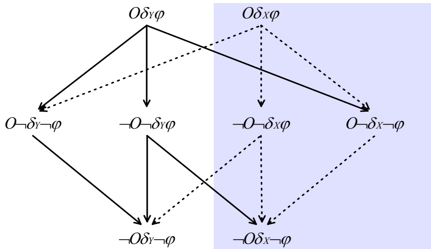
Slika <1.3> «Dijagram snage» za deontičko-prakseološke formule. Osjenjeni
