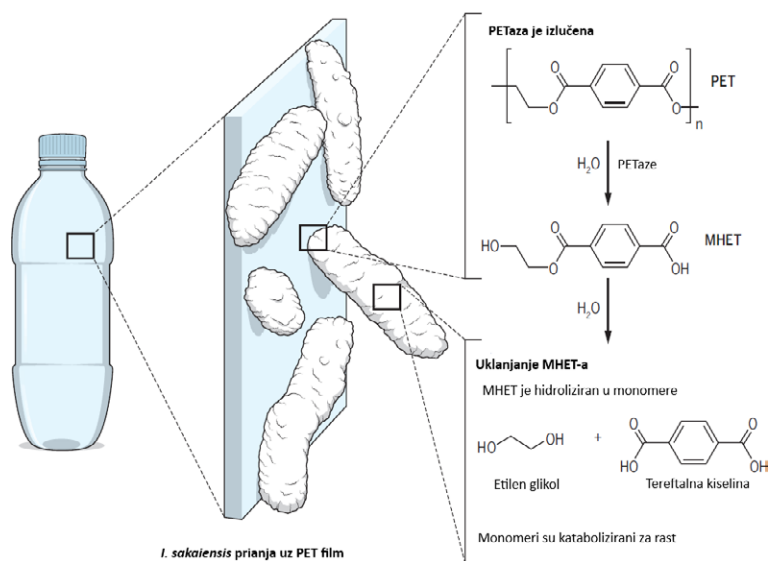
Sl.2 Enzimatska razgradnja PET-a bakterijom I. sakaiensis [115]
