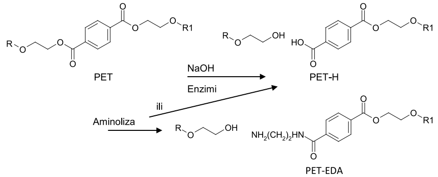
Sl.1 Hidroliza i aminoliza PET-a [45]
